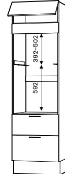
Innbyggingsovn + mikro med 2 store skuffer. Tandembox og Legrabox.
