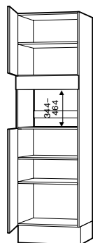
Innbyggingssovn alt mikro
