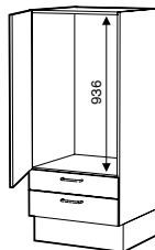
Skap for innbyggings- kjøl/frys med 2 skuffer Tandembox og Legrabox.
