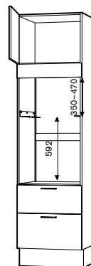
Innbyggingsovn + mikro med 2 store skuffer. Tandembox og Legrabox.
