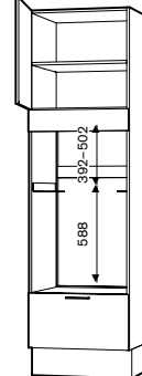
Innbyggingsovn + mikro med skuff. Tandembox og Legrabox.
