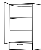
Høyskap for oppvaskmaskin- søyle S med skuff 60 cm. Høyde 105,6 cm. Tandembox og Legrabox.
