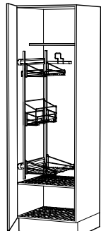
Kosteskap 1 med uttrekkbar innredning og platbelagt bunn 60 cm
