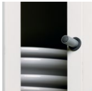
Dørdemper Soft. Lydløs, dempet lukking av skapdøren. Tilbehør som bores inn i skapsiden eller monteres i holdere.
